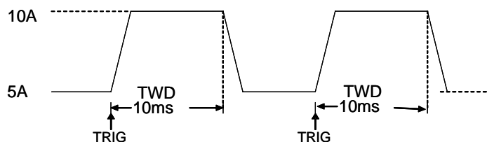
图4.11 脉冲操作模式
