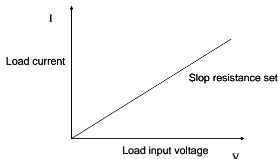
图4.5 定电阻模式
